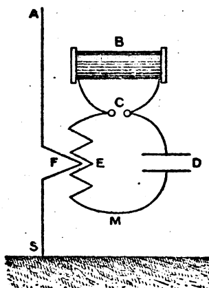
Fig. 8. — Transmetteur Marconi.
