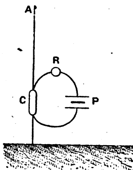
A, antenne. — R, relais faisant fonctionner le Morse. P, pile locale. — C, cohéreur.
