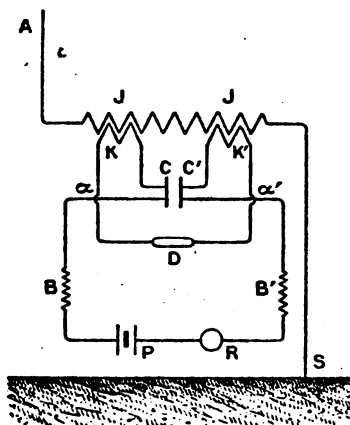
Fig. 9. — Récepteur Marconi.
